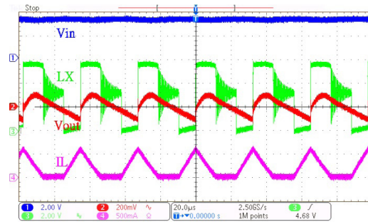
HT7750B 工作 ( I_{OUT}=100mA )
