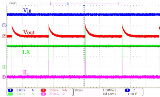
HT7733B 工作 ( I_{OUT}=0mA )
