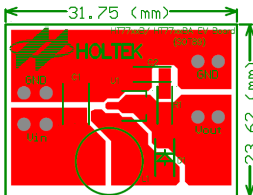
SOT89 PCB 布局范例
