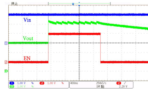
HT7750B 芯片使能
