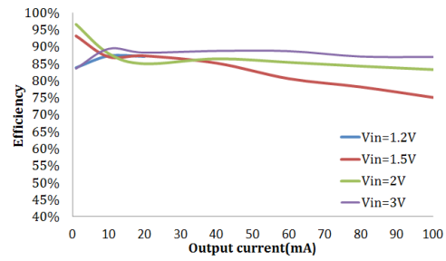
HT7750B 效率 vs. 输出电流
