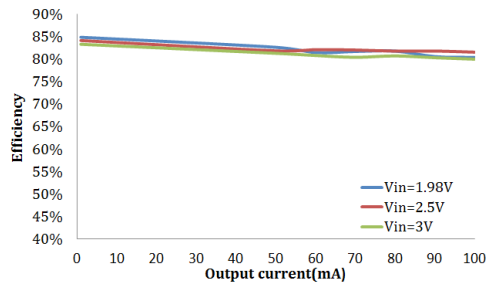
HT7733B 效率 vs. 输出电流
