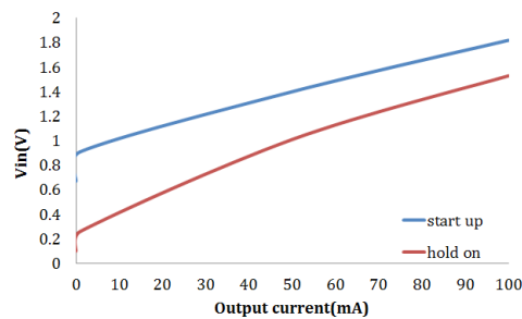
HT7733B 启动 / 保持电压
