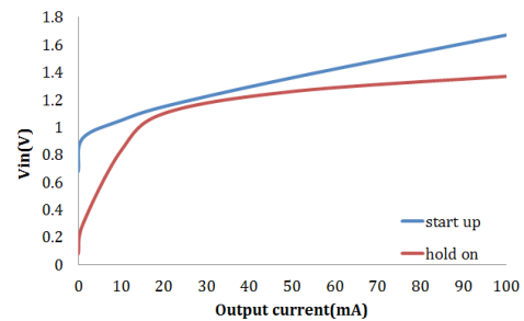
HT7750B 启动 / 保持电压
