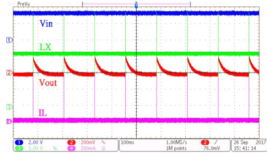
HT7750B 工作 ( I_{OUT}=0mA )
