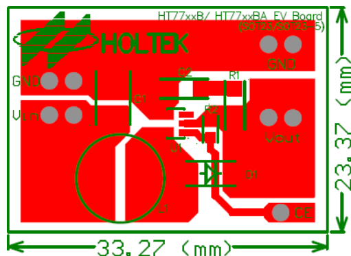
SOT23/SOT23-5 PCB 布局范例
