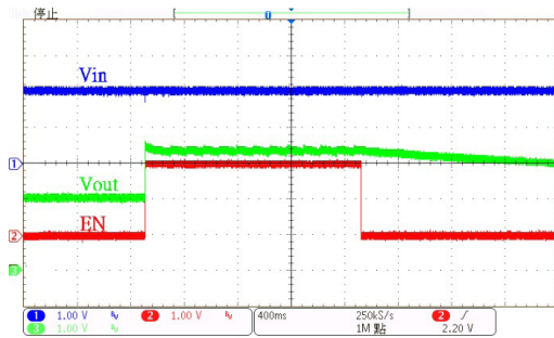
HT7733B 芯片使能
