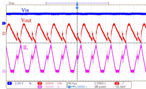
HT7733B 工作 ( I_{OUT}=100mA )
