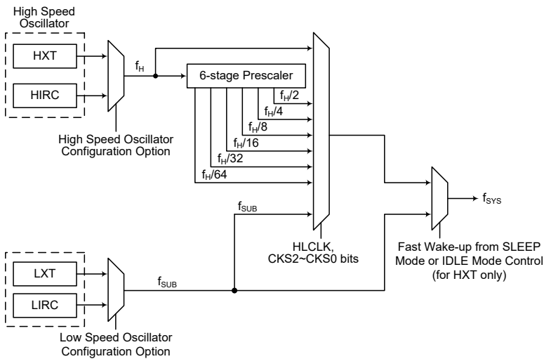
系统时钟配置
