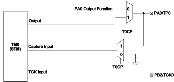
TM0 功能引脚控制方框图
