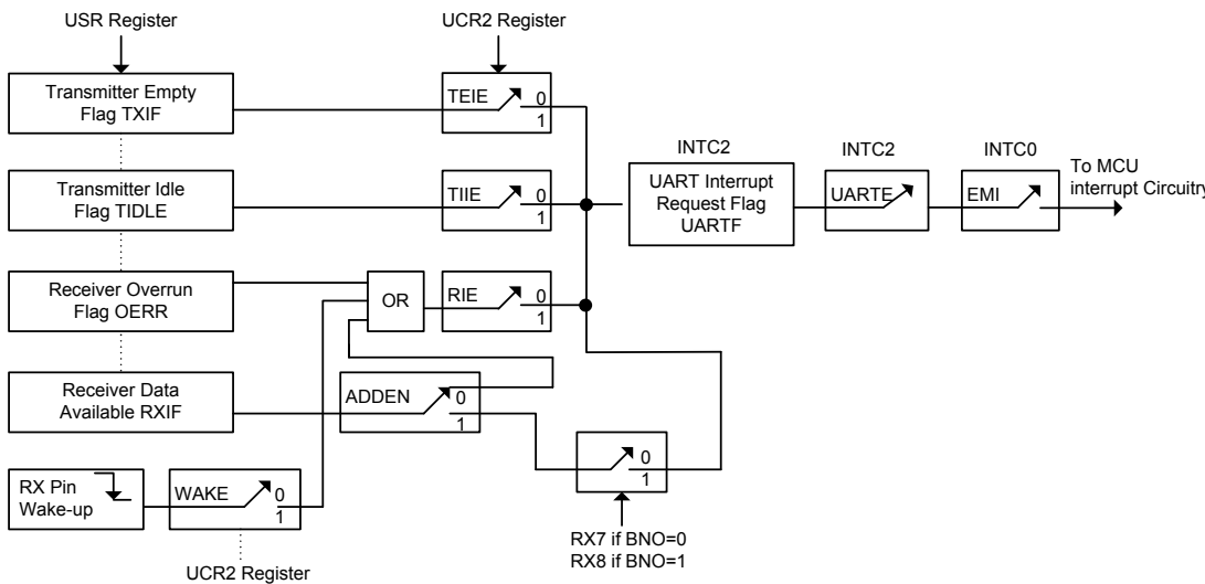
UART 中断结构
