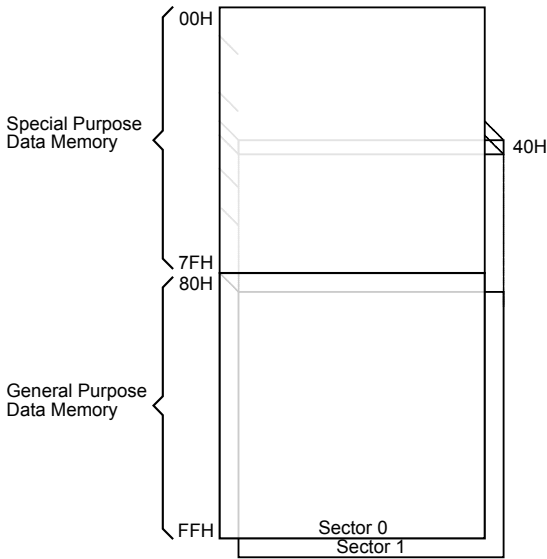
数据存储器结构
