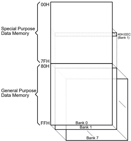
数据存储器结构
