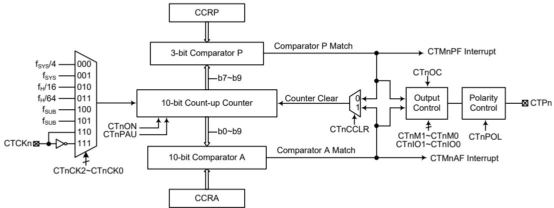
简易型 TM 方框图 (n=0~1)
