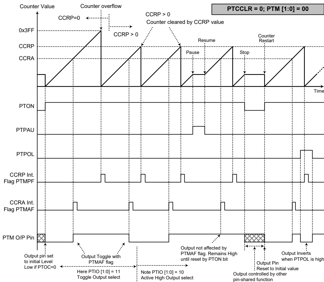
比较器匹配输出模式 – PTCCLR=0
