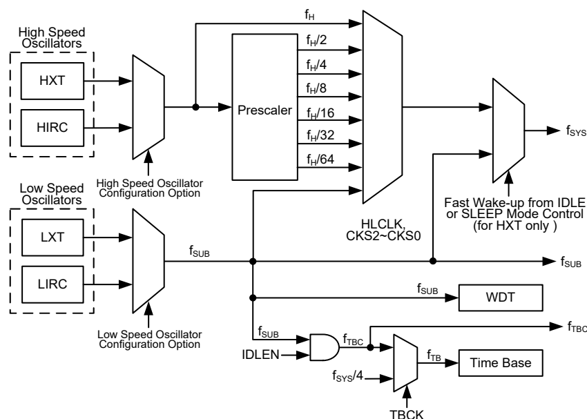
单片机时钟配置
