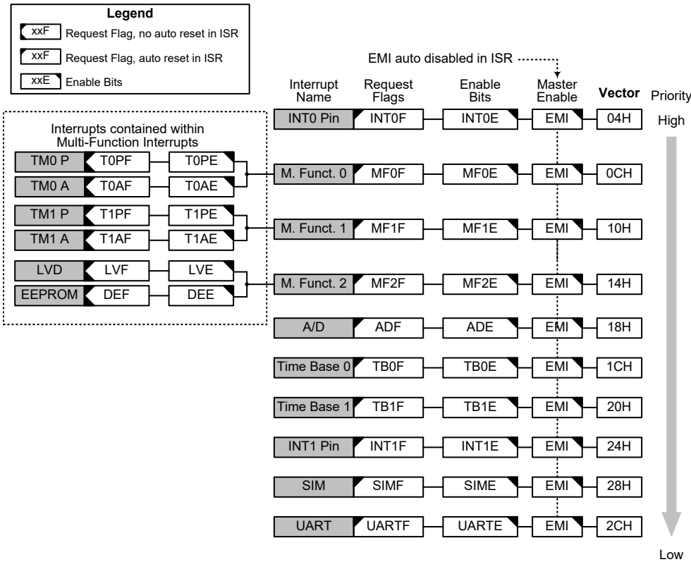
中断结构
