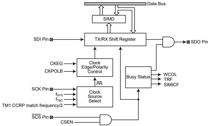
SPI 方框图
