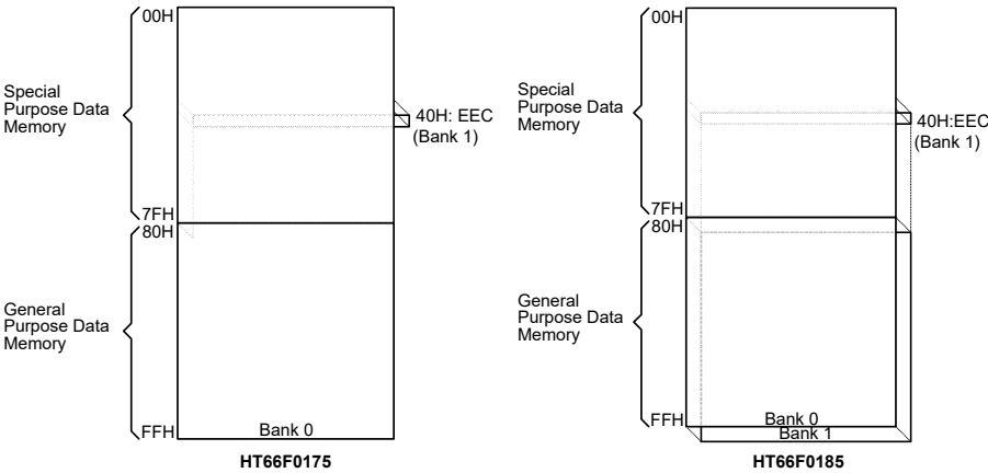
数据存储器结构
