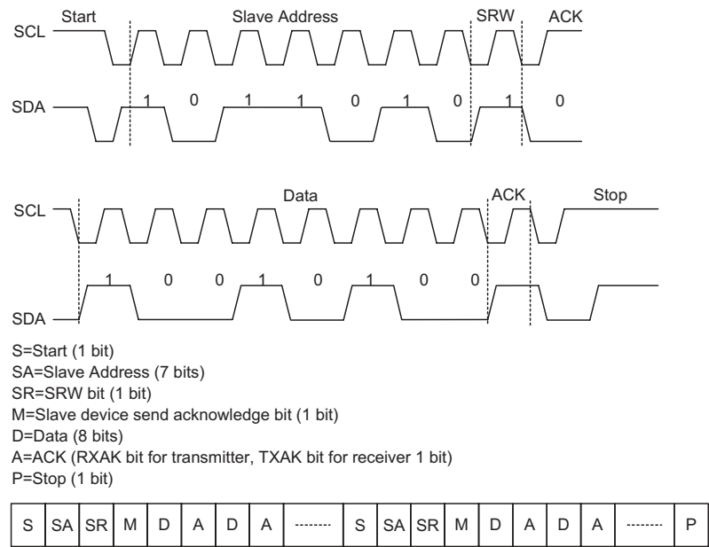
I 2 C 通信时序图
