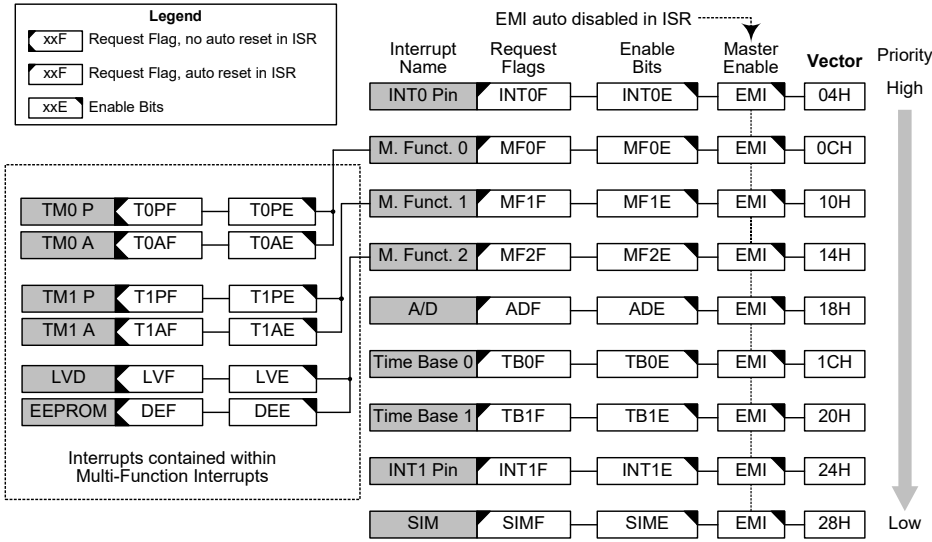
中断结构 – HT66F0175
