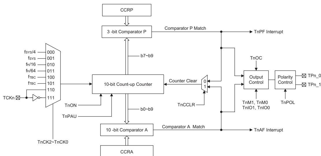
简易型 TM 方框图 (n=0 或 1)
