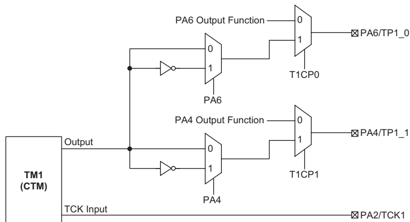
TM1 功能引脚控制方框图
