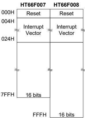
程序存储器结构
