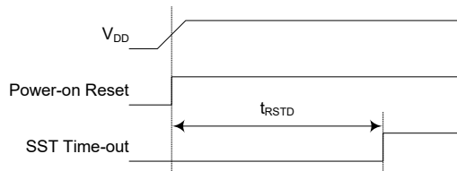
上电复位时序图
