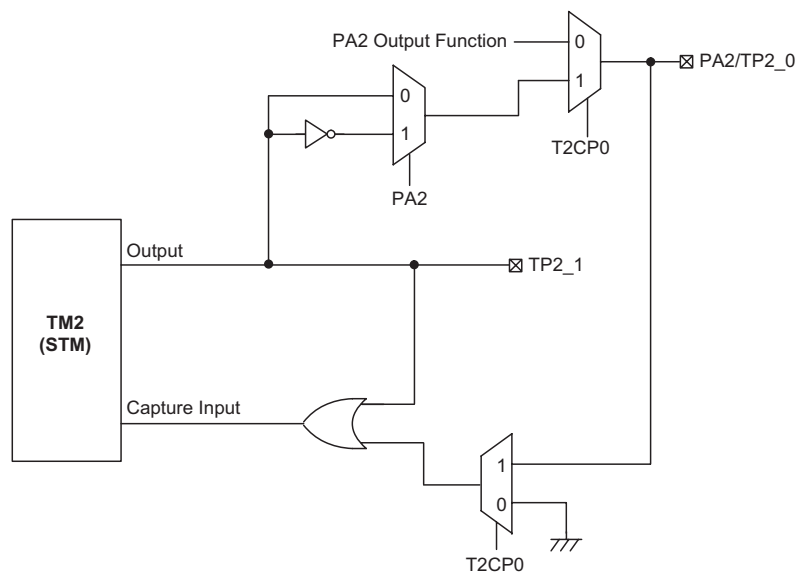
TM2 功能引脚控制方框图
