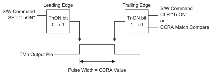
单脉冲产生示意图 (n=2)
