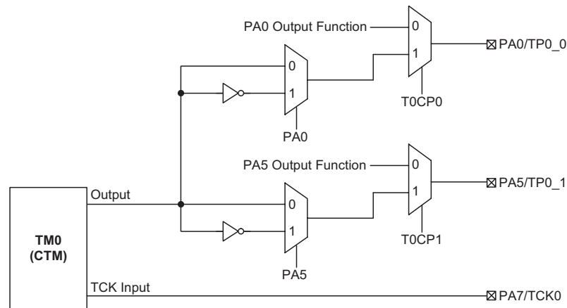
TM0 功能引脚控制方框图
