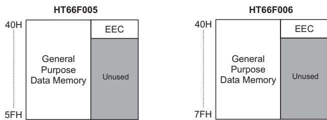
通用数据存储器
