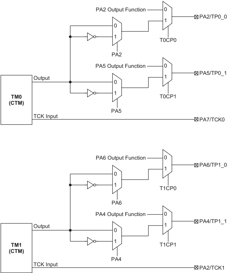
HT66F005/HT66F006 TM 功能引脚控制方框图
