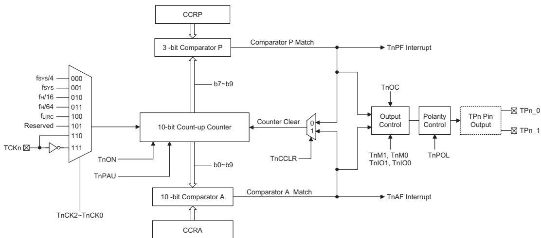
简易型 TM 方框图 (n=0, 1)
