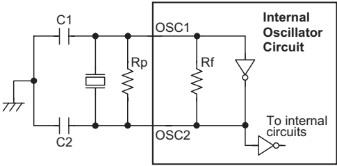
晶体 / 陶瓷振荡器 – HXT
