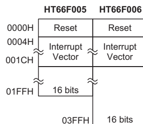
程序存储器结构
