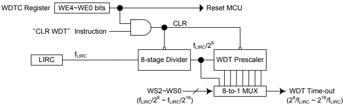
看门狗定时器
