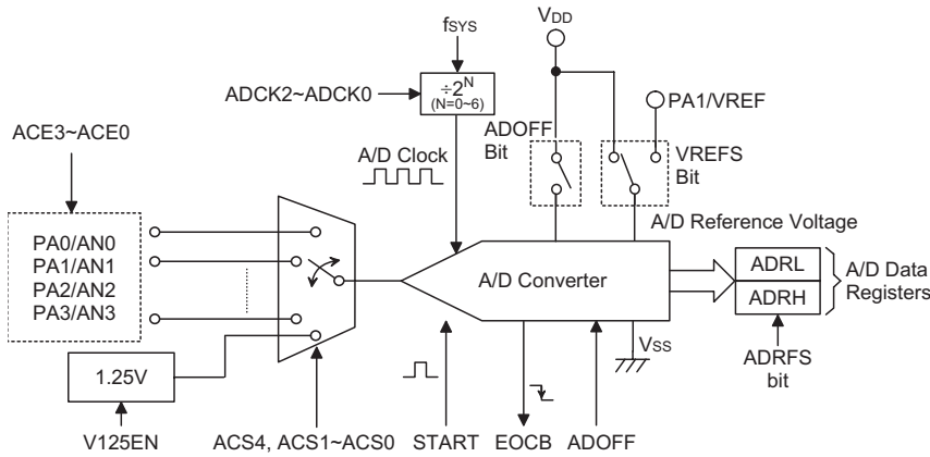
A/D 转换器结构
