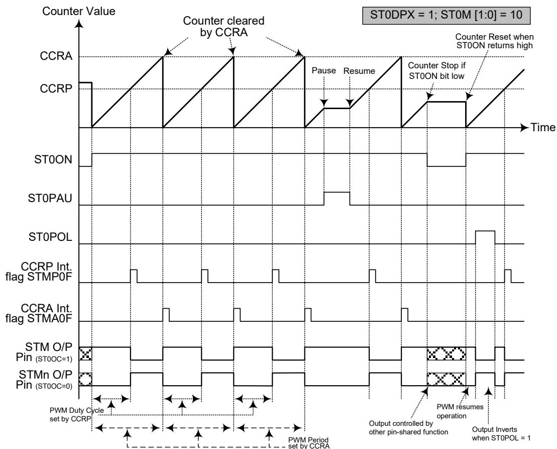
PWM 输出模式 – ST0DPX=1
