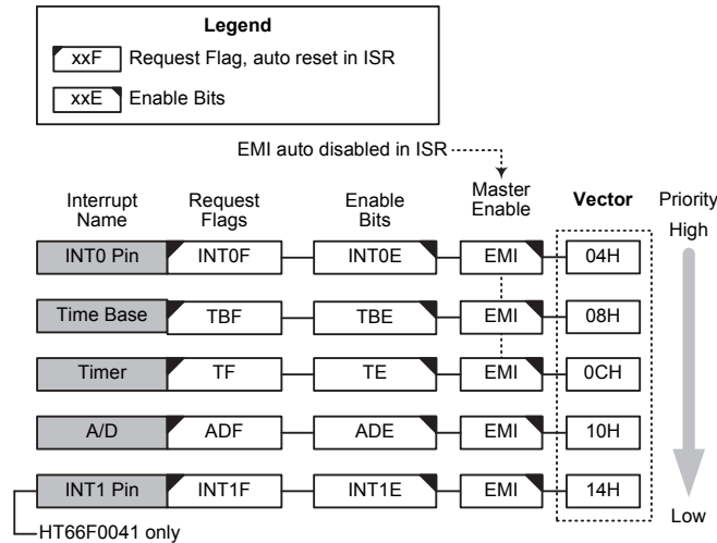
中断结构
