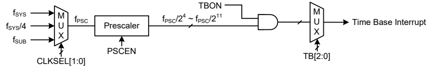
时基中断
