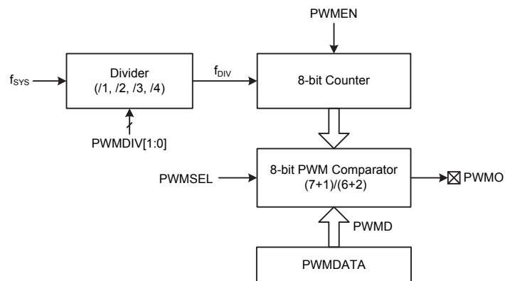
PWM 方框图
