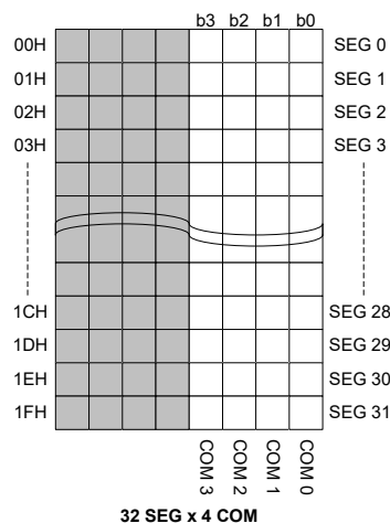
BS67F350 LCD 存储器映射图
