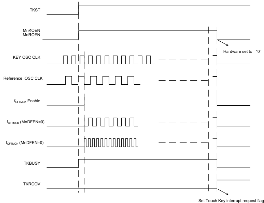
触控按键手动扫描时序图
