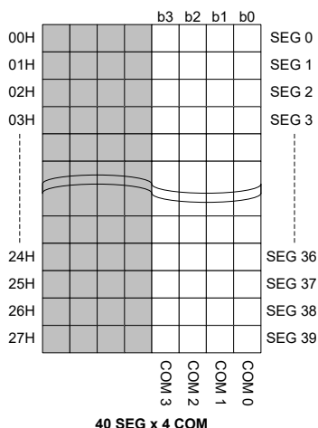
BS67F360 LCD 存储器映射图
