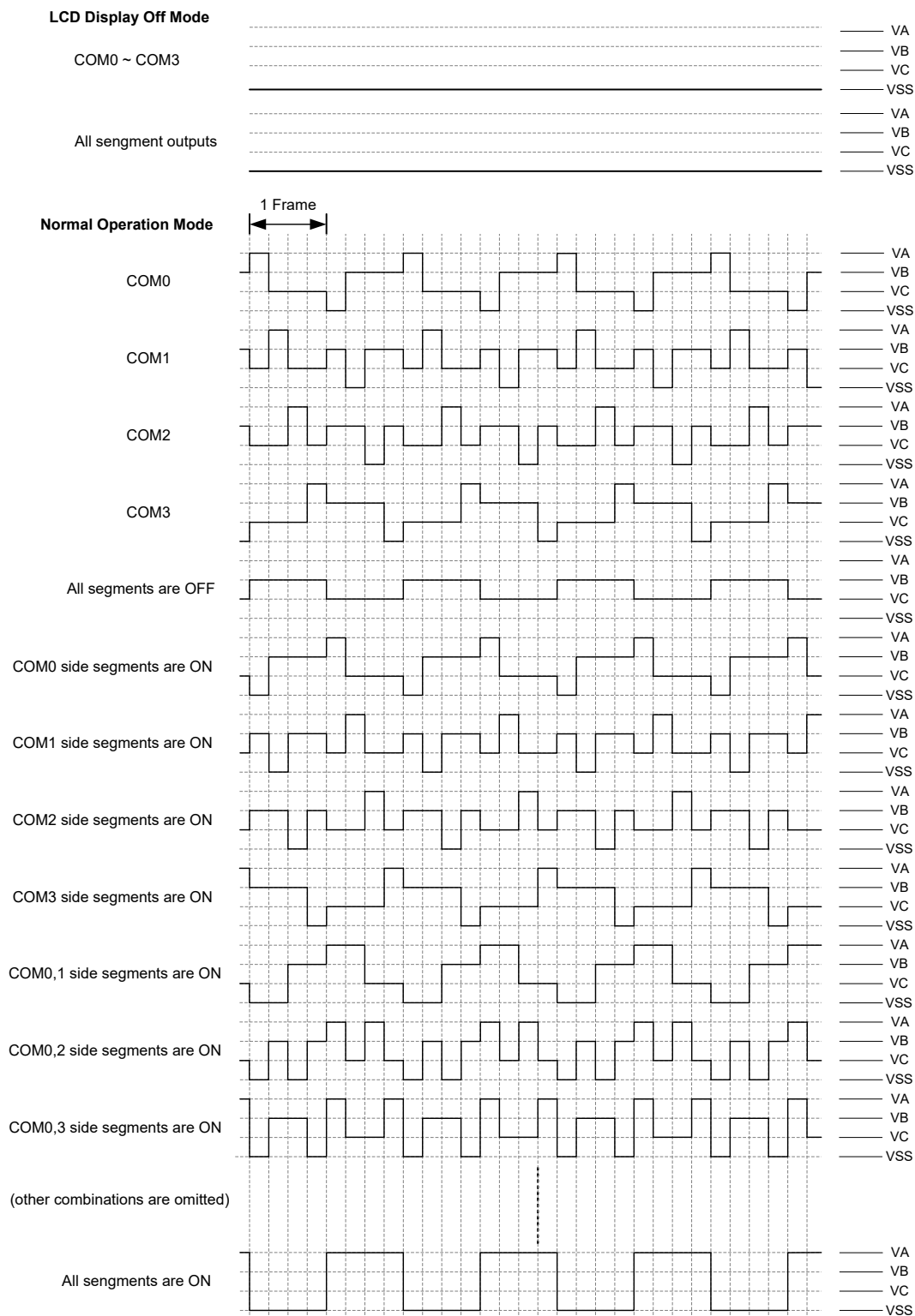
LCD 驱动输出 – B 型 , 1/4 Duty, 1/3 Bias
