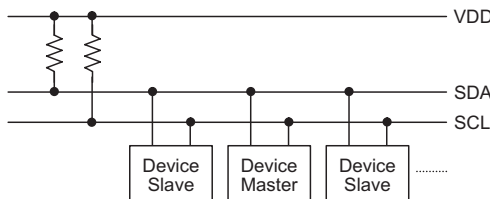
I 2 C 主从总线连接图
