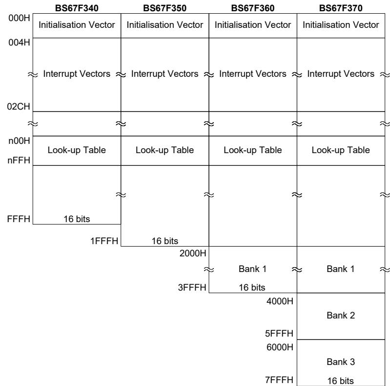
程序存储器结构
