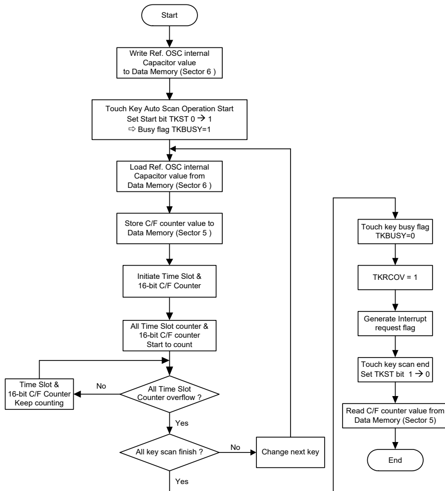
自动扫描模式流程图 – TKMOD=0, TSCS=0
