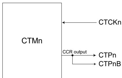
CTM 功能引脚控制框图 -n=0 或 1
