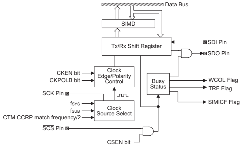
SPI 方框图
