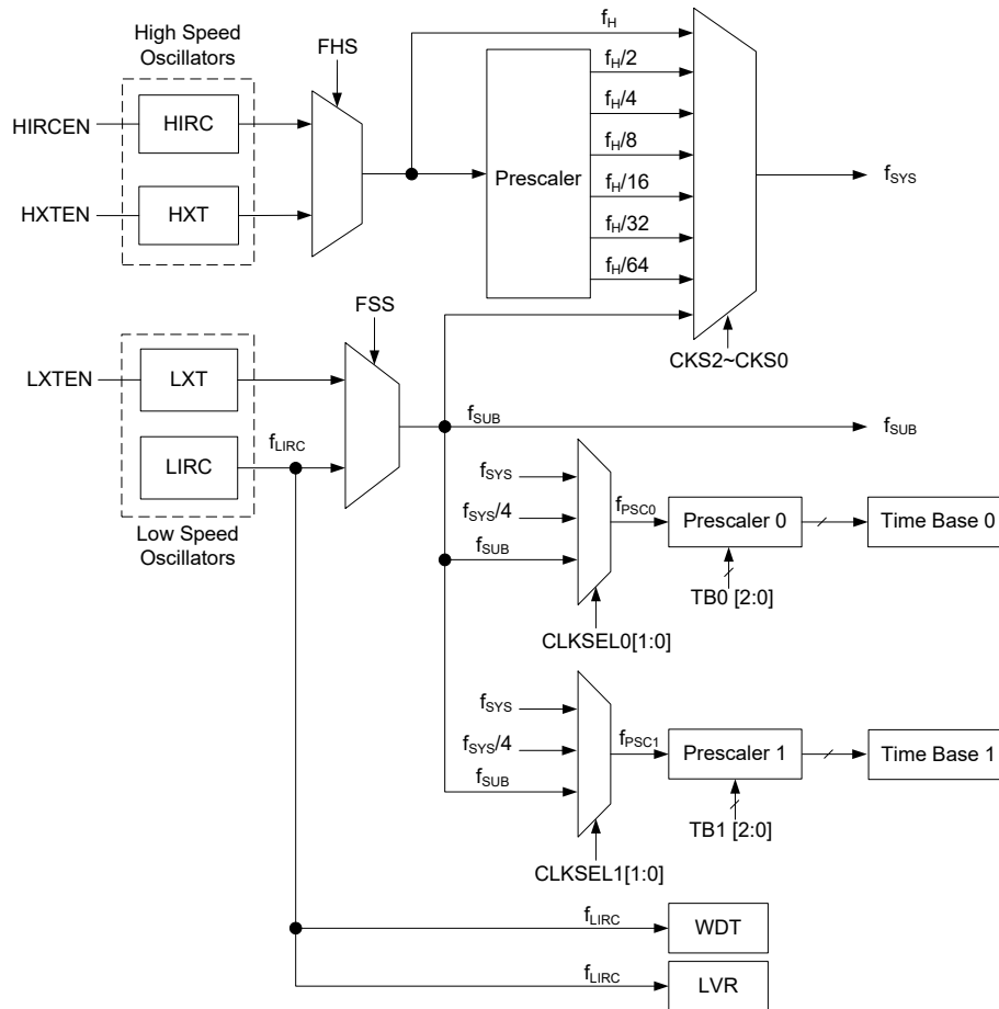
单片机时钟配置
