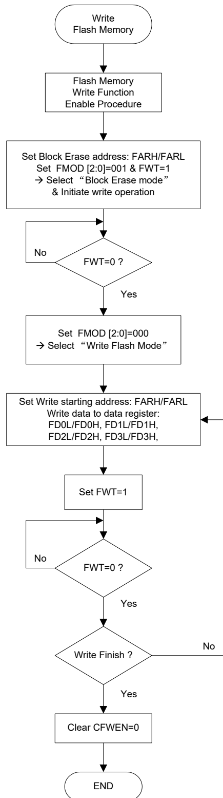
写 Flash 存储器步骤 – BS67F340
