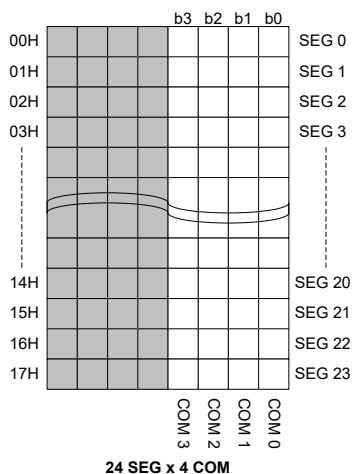
BS67F340 LCD 存储器映射图
