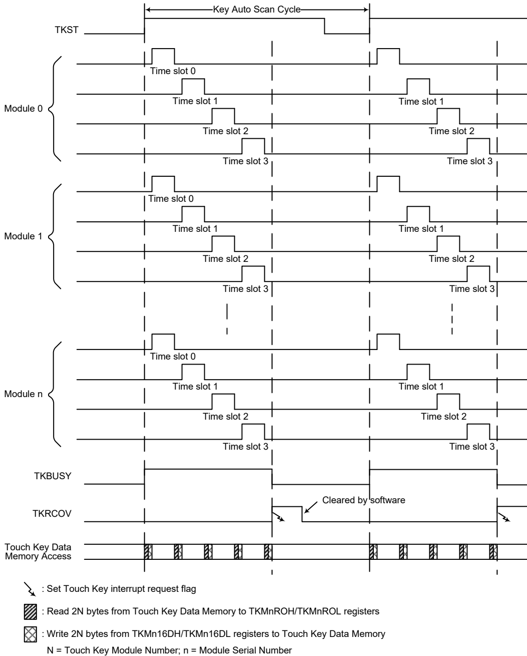
触控按键自动扫描时序图
