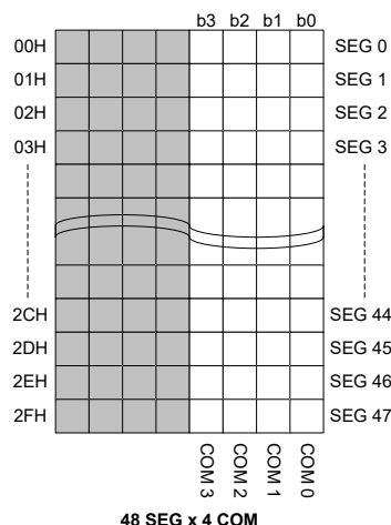
BS67F370 LCD 存储器映射图
