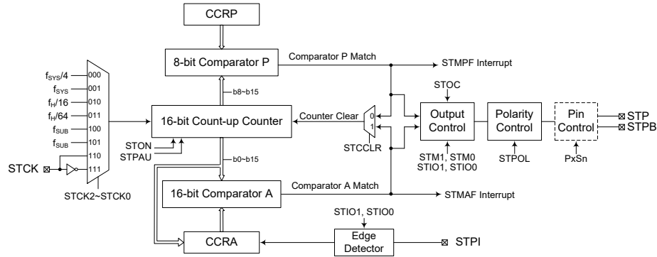
标准型 TM 框图
