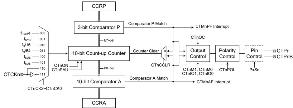
简易型 TM 方框图 – n=0 或 1
