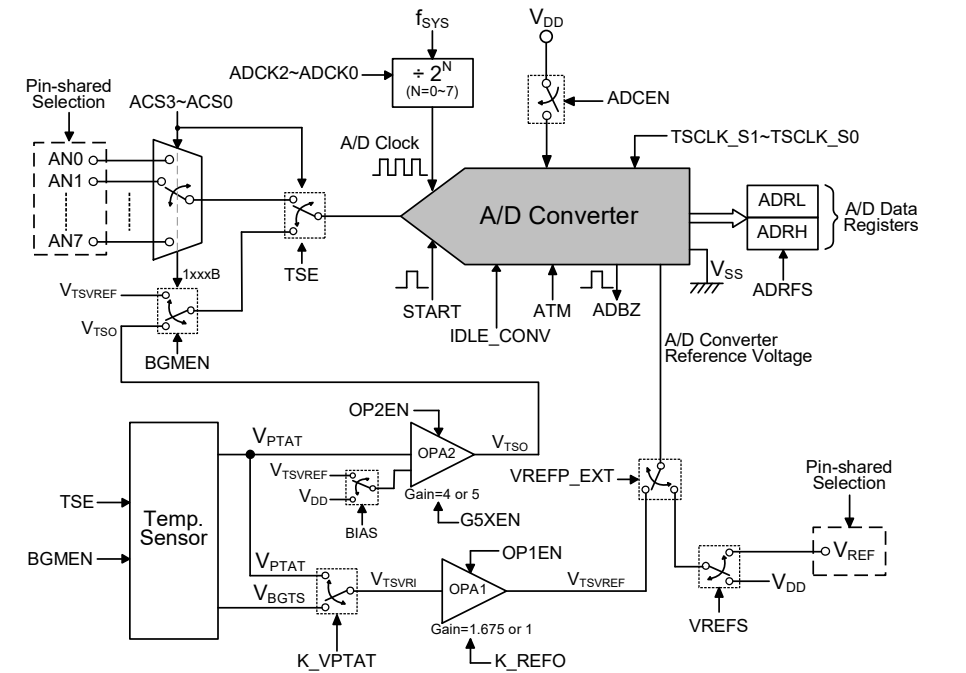
带温度传感器的 A/D 转换器结构
