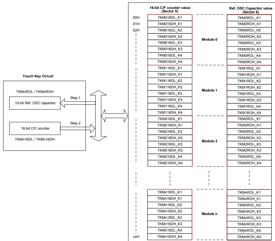
触控按键模块数据存储器分布
