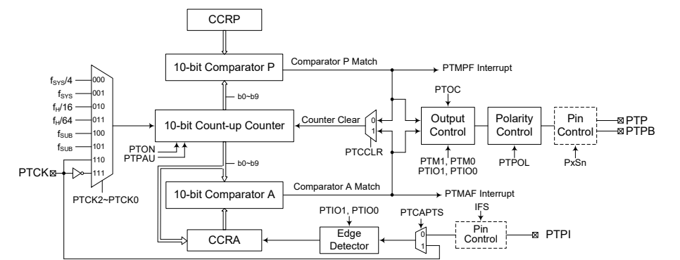
周期型 TM 方框图
