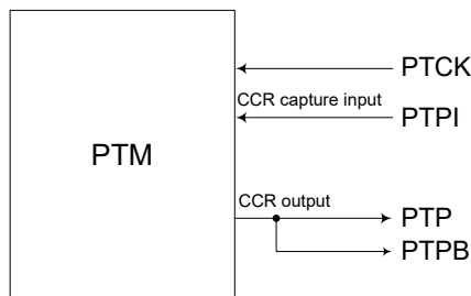
PTM 功能引脚控制框图
