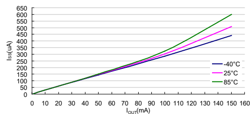
I_{SS} vs I_{OUT} : HT75C0-7 ( V_{IN}=14V )
