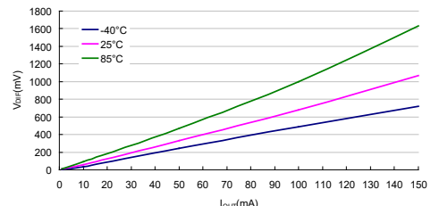
压差：HT75C0-7
