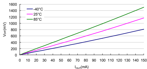
压差：HT7560-7
