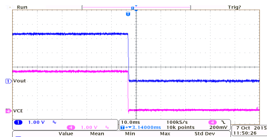
开关响应: HT7533-7 ( I_{OUT}=100mA , V_{CE}=2.7V to 0V)
