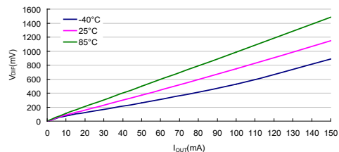
压差：HT7550-7
