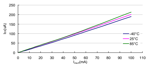
I_{SS} vs I_{OUT} : HT7533-7 ( V_{IN}=5.3V )
