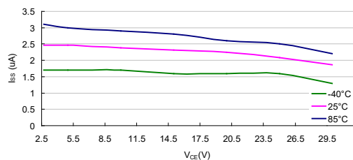
I_{SS} vs V_{CE} : HT7533-7 ( I_{OUT}=0mA )
