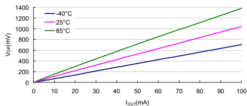
压差：HT7533-7
