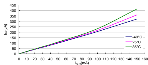
I_{SS} vs I_{OUT} : HT7550-7 ( V_{IN}=7.0V )
