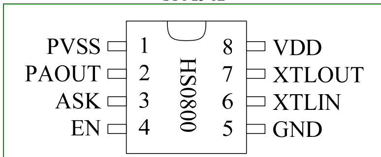
SOP 8
