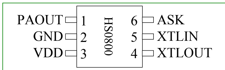
SOT 23-6L
