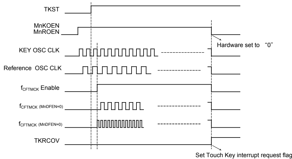
触控按键扫描模式时序图
