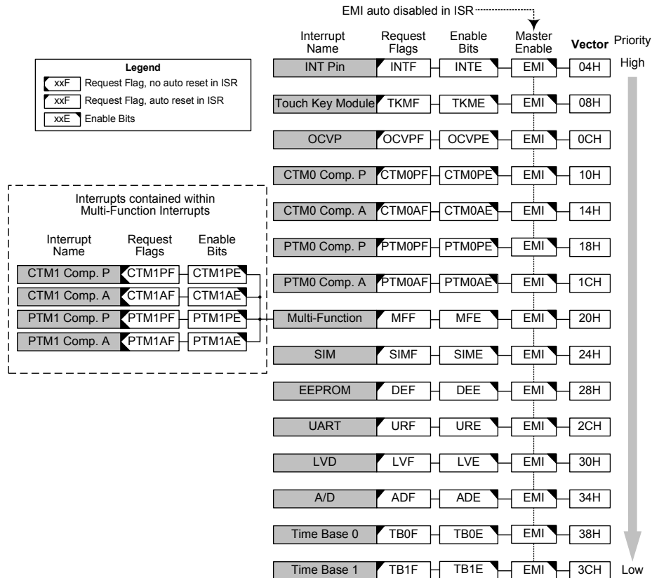
中断结构 – BS87D20A-3
