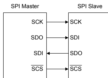
SPI 主机 / 从机连接
