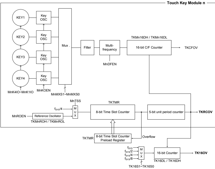
触控按键结构
