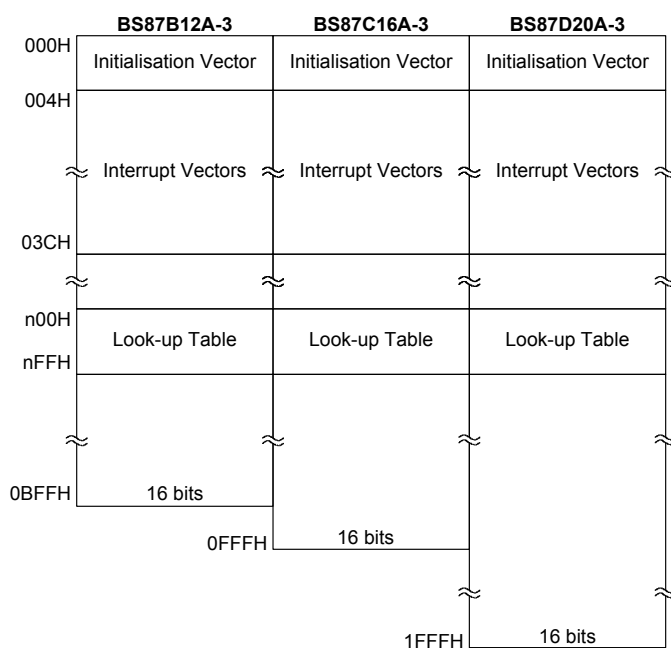
程序存储器结构
