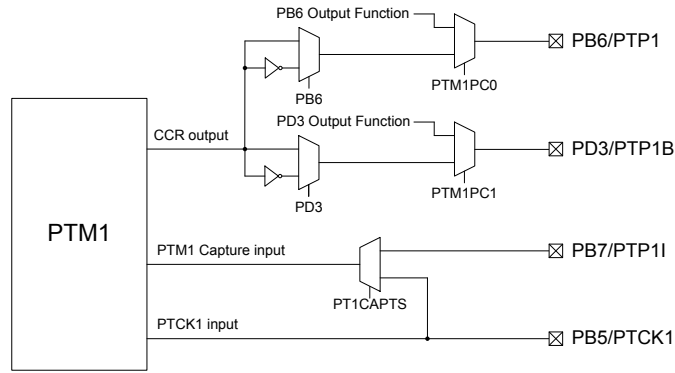
PTM1 功能引脚控制方框图 – BS87C16A-3 & BS87D20A-3
