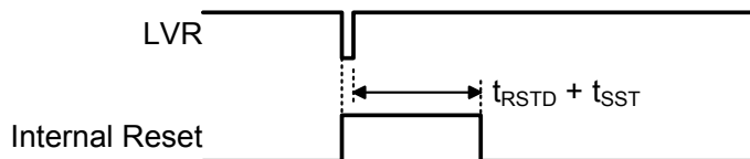
低电压复位时序图
