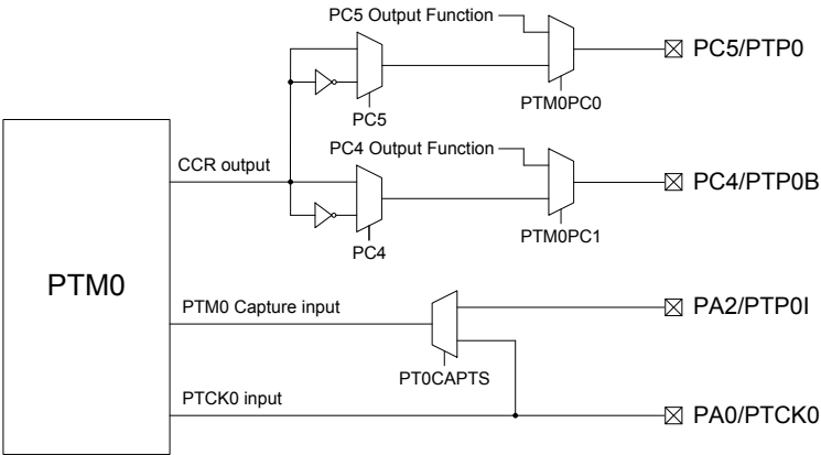
PTM0 功能引脚控制方框图
