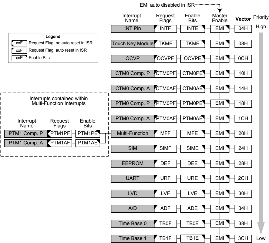
中断结构 – BS87C16A-3
