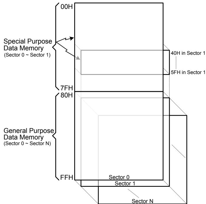
数据存储器结构
