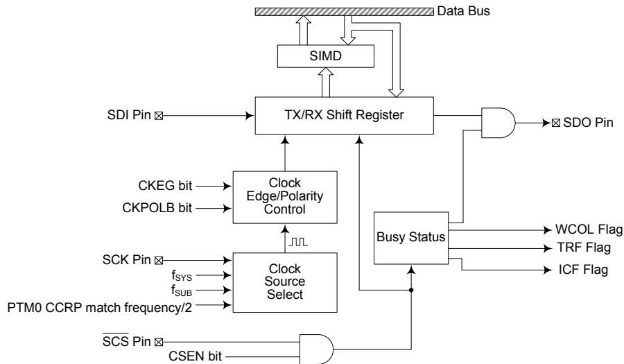
SPI 方框图
