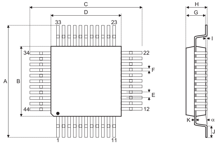
44-pin LQFP (10mm×10mm) (FP2.0mm) 外形尺寸
