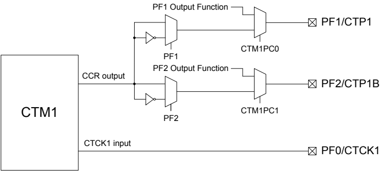
CTM1 功能引脚控制方框图 – BS87D20A-3
