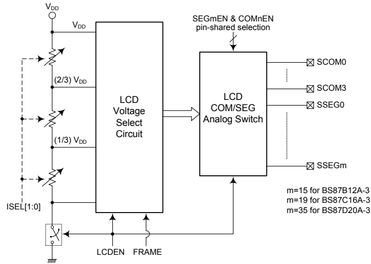
软件控制 LCD 驱动结构
