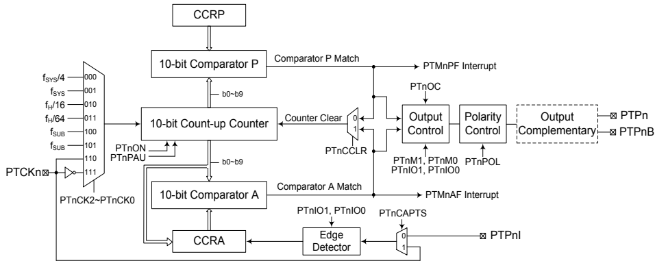
10-bit 周期型 TM 方框图 – n=0 或 1
