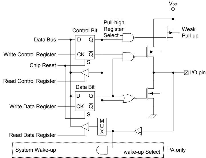
通用输入 / 输出端口结构
