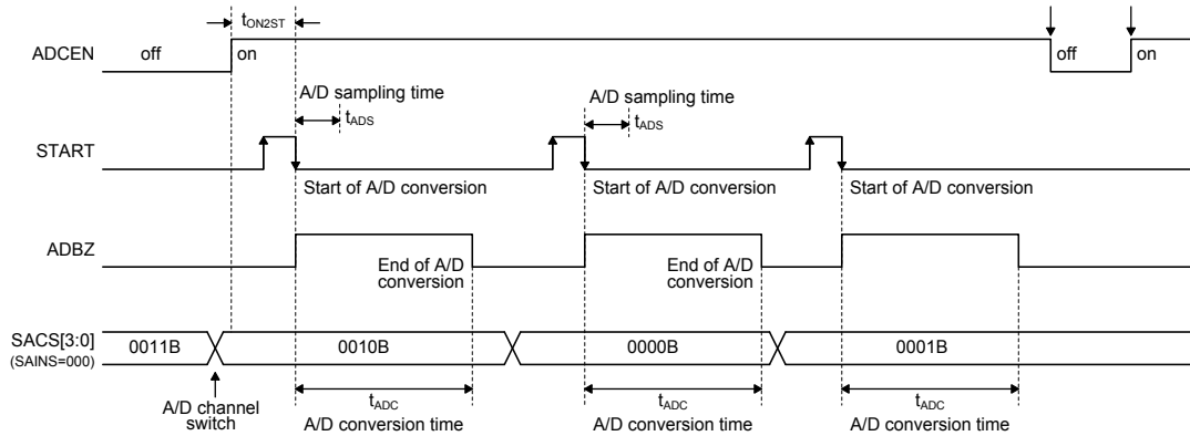
A/D 转换时序 – 外部通道输入
