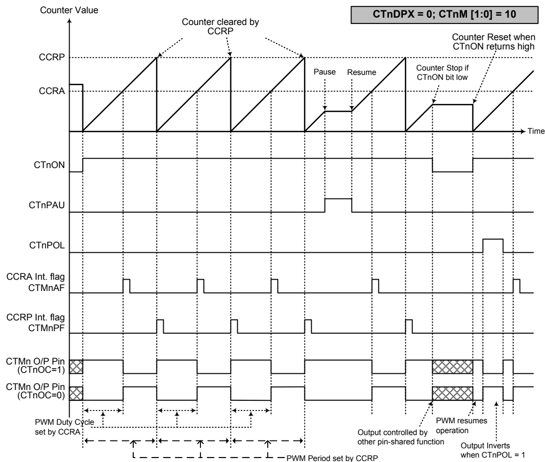
PWM 输出模式 – CTnDPX=0
