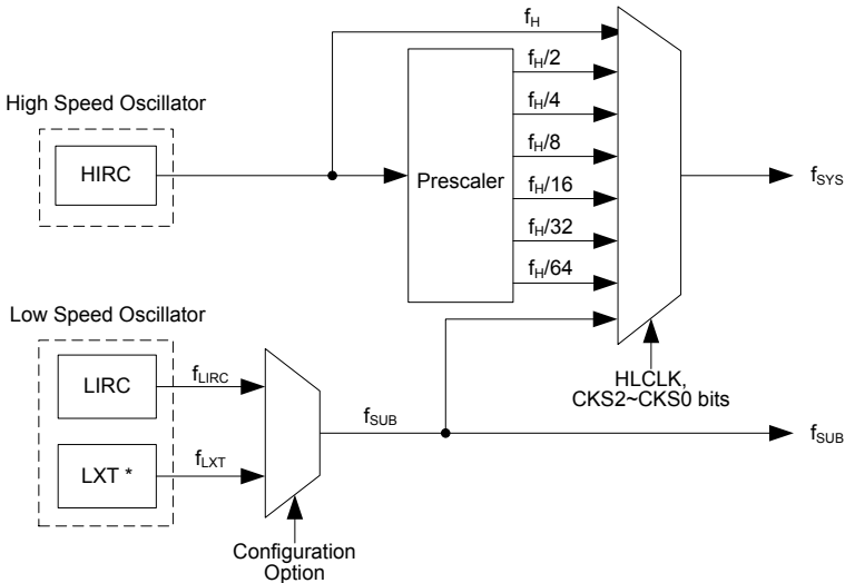
系统时钟配置
