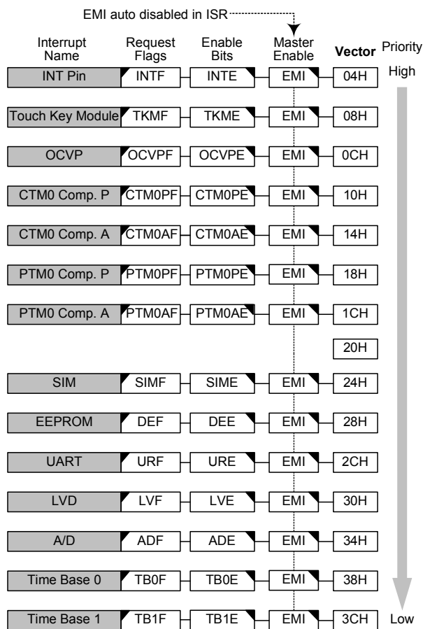
中断结构 – BS87B12A-3
