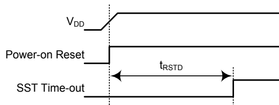
上电复位时序图
