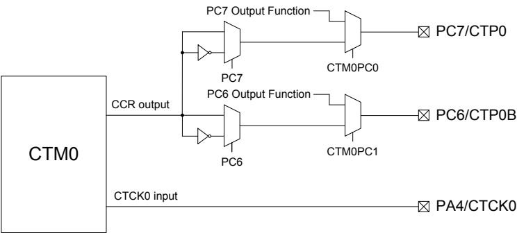
CTM0 功能引脚控制方框图
