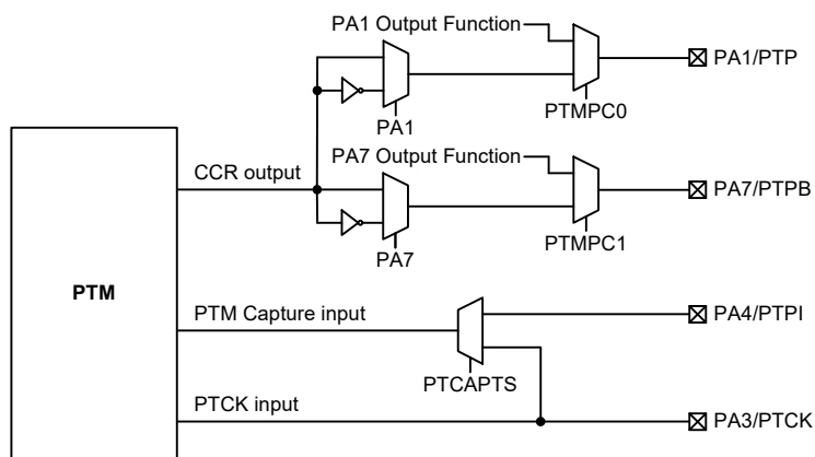
PTM 功能引脚控制方框图
