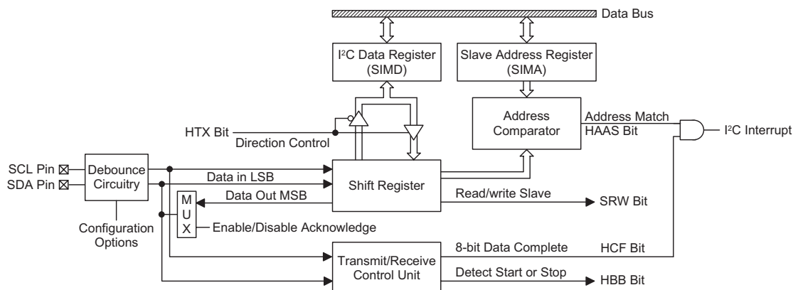
I²C 方框图
