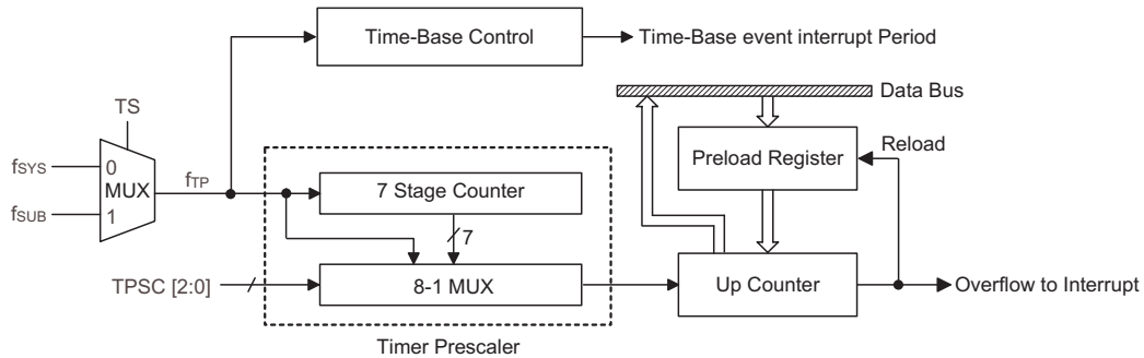
定时 / 计数器
