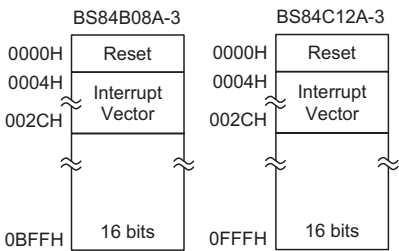
Flash 程序存储器结构
