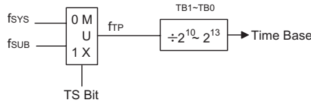
时基结构
