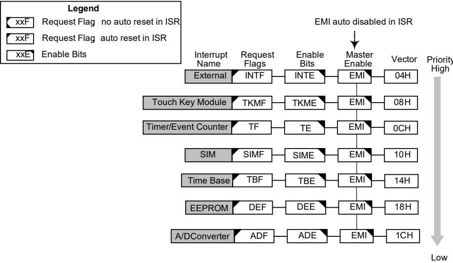
中断结构
