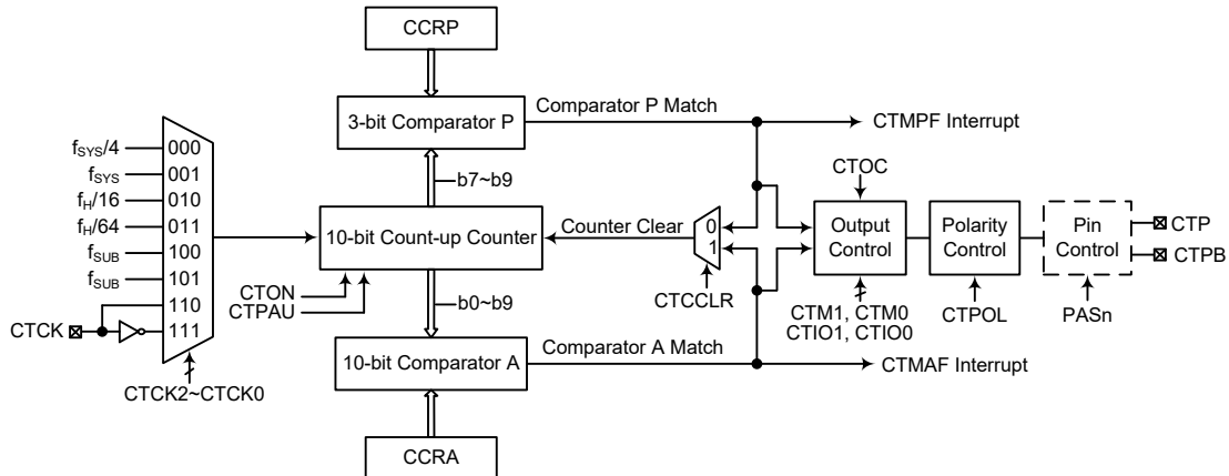
简易型 TM 方框图
