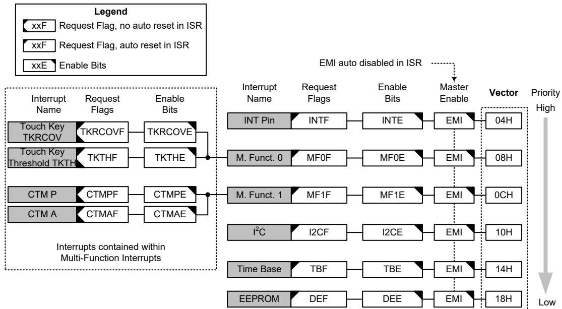
中断结构 – BS83B04L
