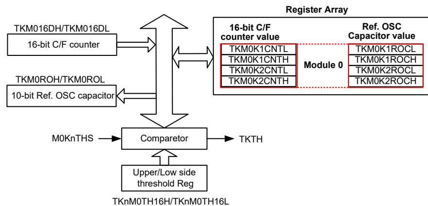
触控按键寄存器分布
