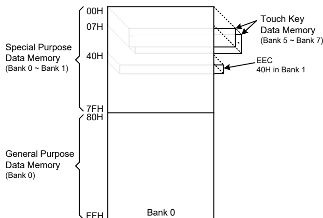
数据存储器结构 – BS83B04L
