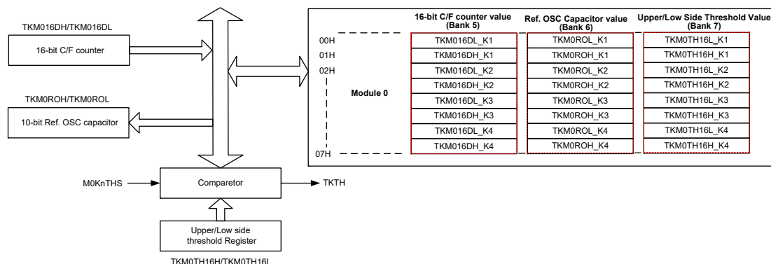
触控按键寄存器分布
