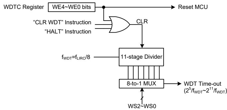
看门狗定时器
