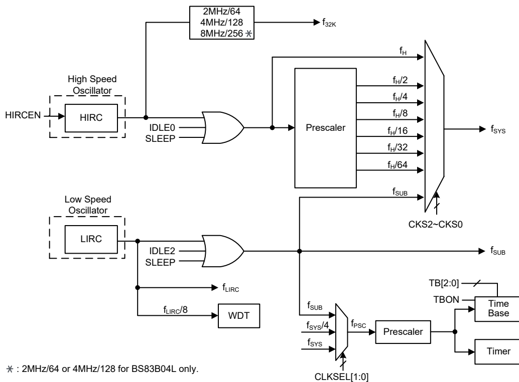
单片机时钟配置
