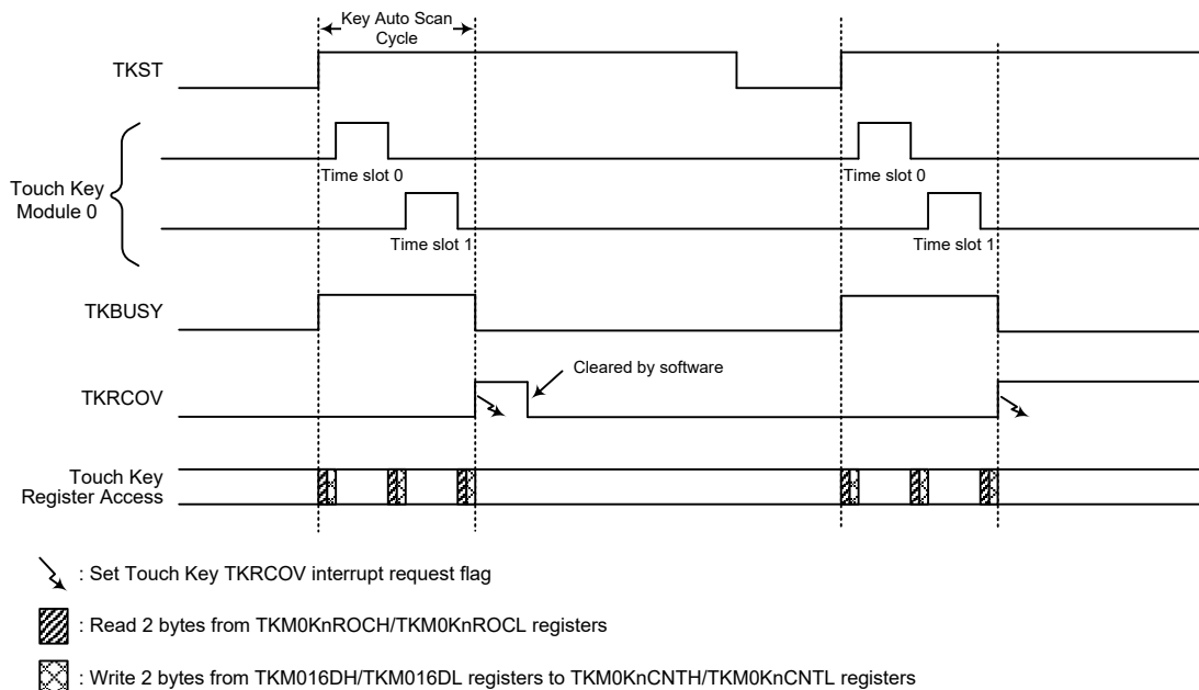
触控按键自动扫描模式时序图
