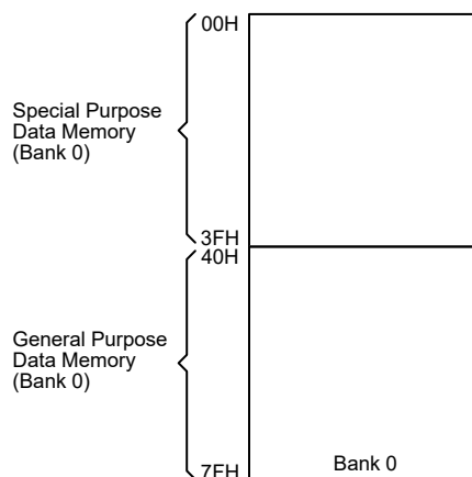
数据存储器结构 – BS83A02L
