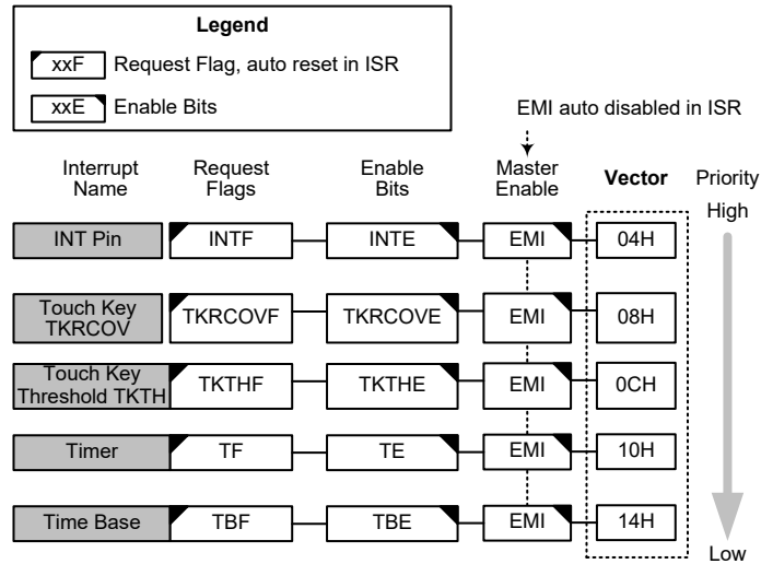
中断结构 – BS83A02L
