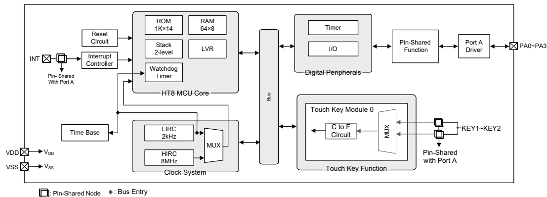
BS83A02L
