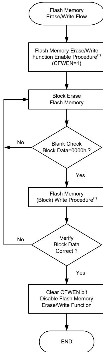
Flash 存储器擦 / 写流程 – BS66F340C
