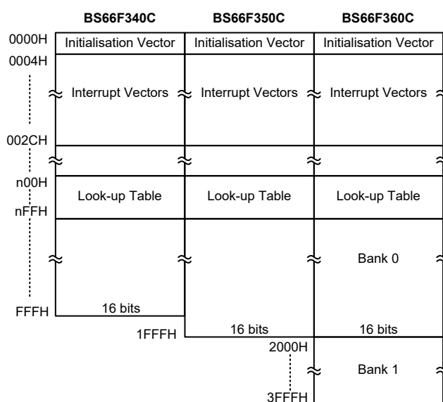
程序存储器结构
