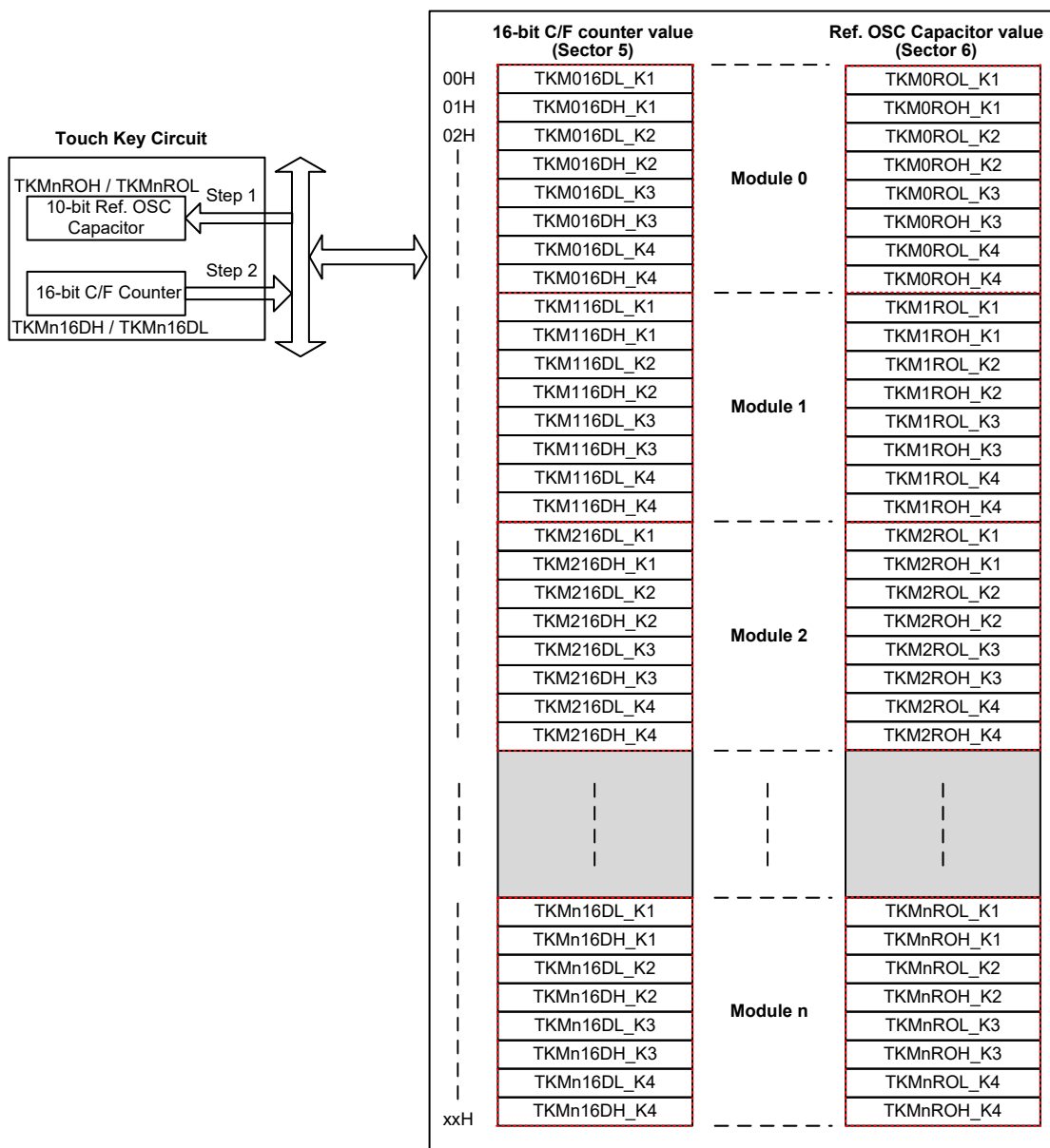
触控按键模块数据存储分布
