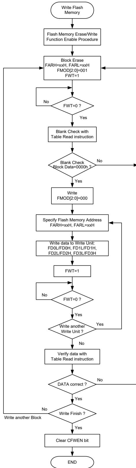
Flash 存储器写流程 – BS66F340C
