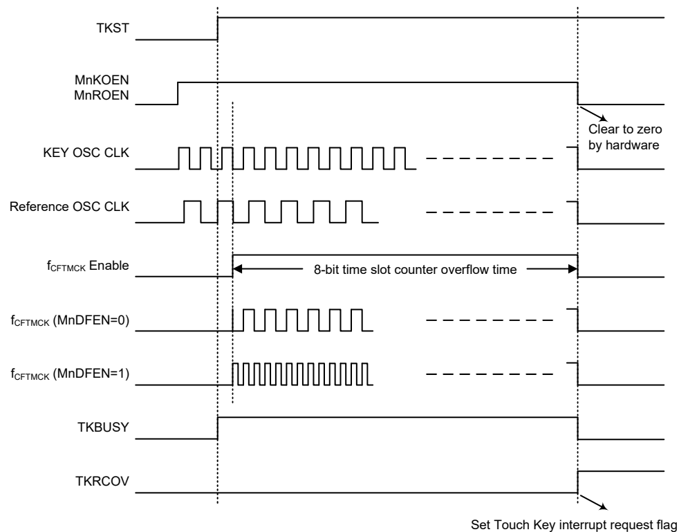
触控按键手动扫描时序图
