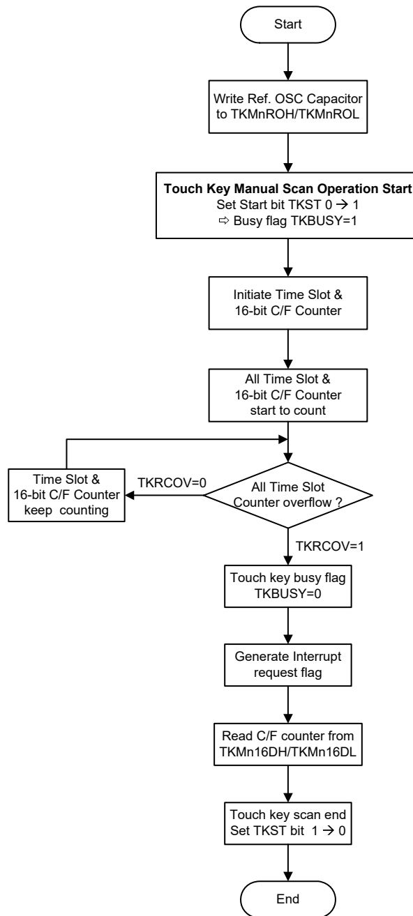
触控按键手动模式流程图 – TKMOD=1, TSCS=0
