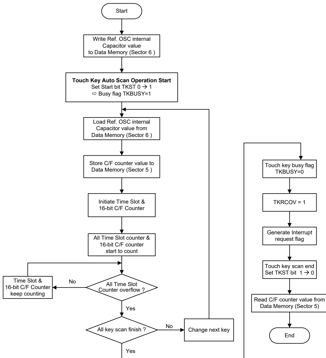
触控按键自动扫描模式流程图 – TKMOD=0, TSCS=0
