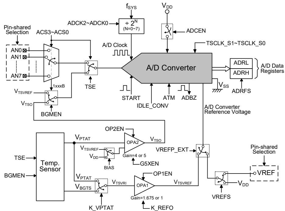
带温度传感器的 A/D 转换器结构
