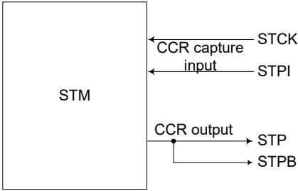
STM 功能引脚控制框图
