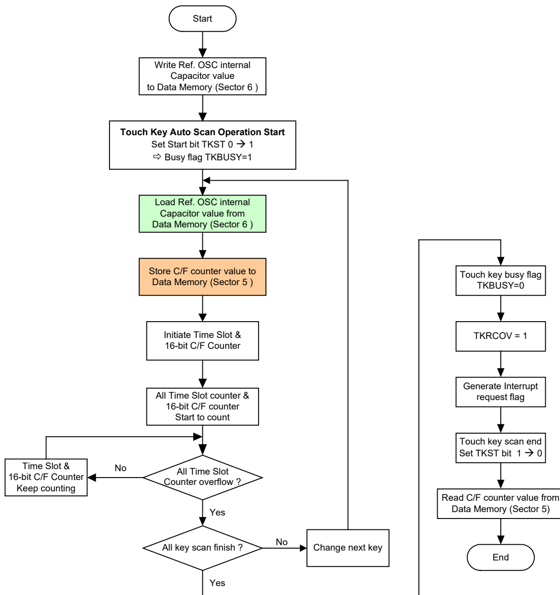
自动扫描模式流程图— TKMOD=0, TSCS=0
