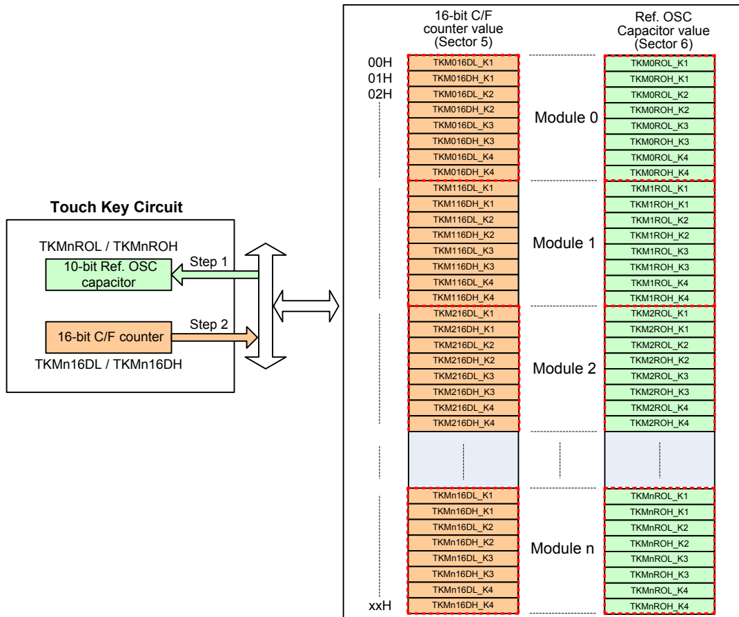
触控按键模块数据存储区分布
