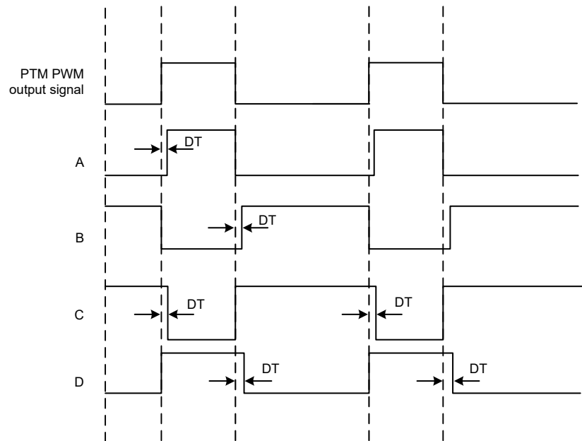
带死区时间控制的互补 PWM 输出
