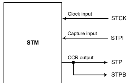
STM 功能引脚控制方框图
