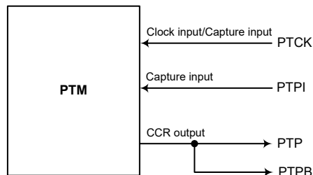
PTM 功能引脚控制方框图
