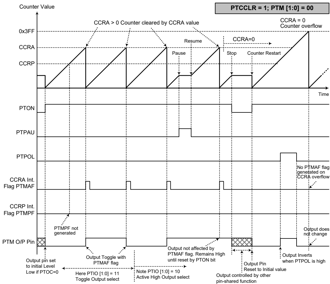
比较器匹配输出模式 – PTCCCLR=1
