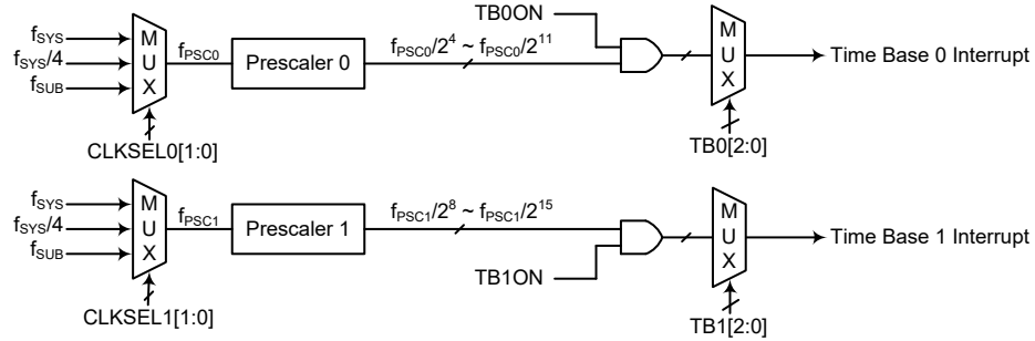
时基中断
