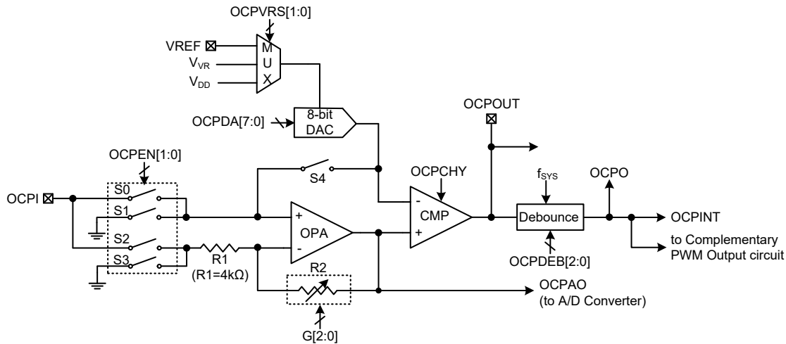
OCP 电路方框图
