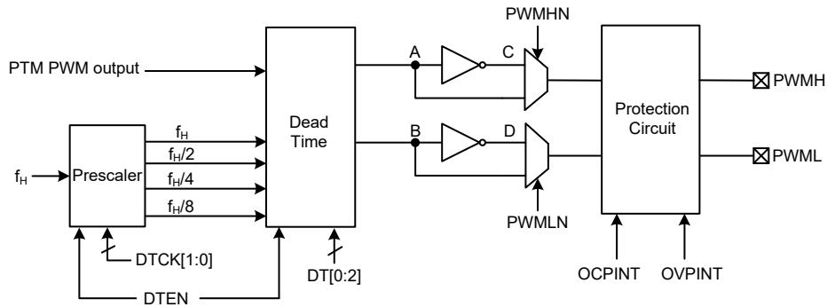
带死区时间的互补 PWM 输出方框图
