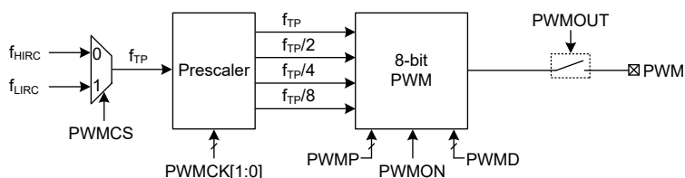
PWM 方框图
